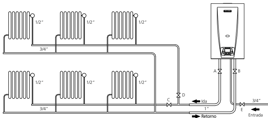
FIG. 5 Instalación para calefacción por radiadores
